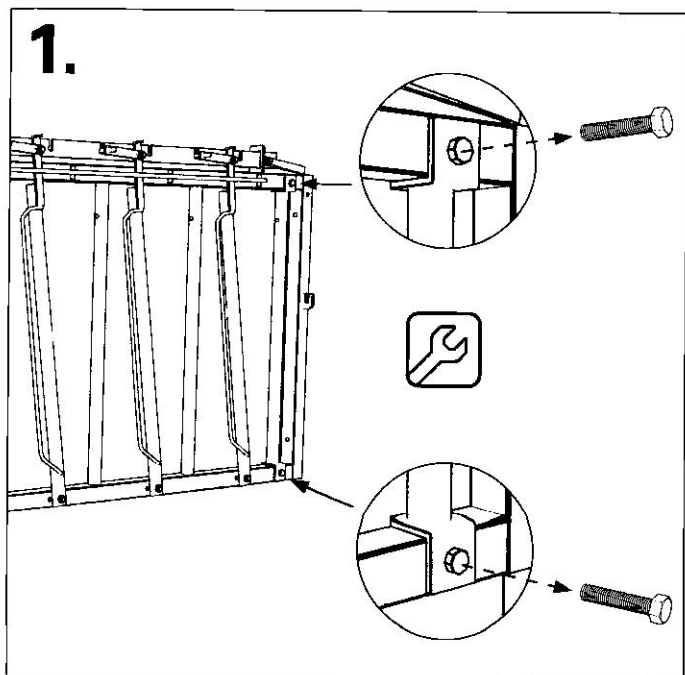
8x M10 x 130
